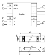
Scheda tecnica Philips HF-Ri TD 2 28-54 TL5 E+ 195-240V
