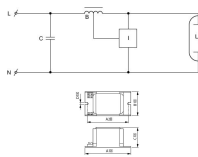
Scheda tecnica Philips HID-HeavyDuty BSN 400 L33-TS 230V 50Hz HD3-166 Descarga
